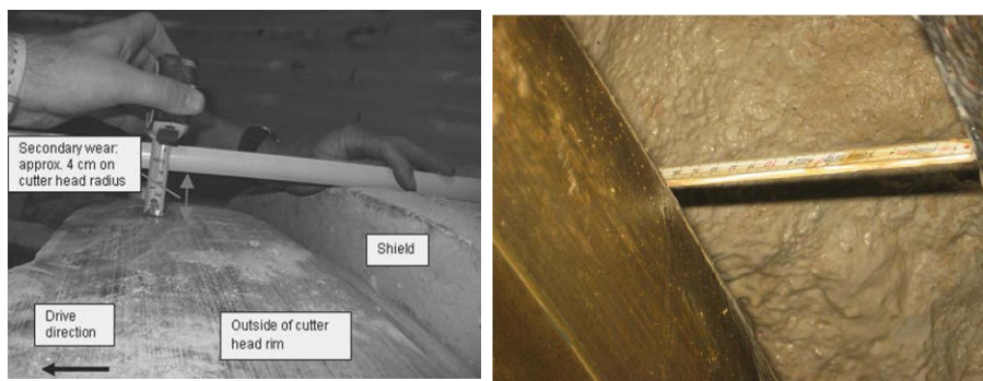
شکل ۲. سایش ثانویه شدید در حد فاصل پشت کله حفار و سپر یک ماشین حفاری مکانیزه از نوع فشار تعادلی خاک [۸] شکل ۳. سایش ثانویه زیاد در دیواره خارجی کله حفار یک ماشین EPB با قطر حفاری ۴/۷ متر [۷]
