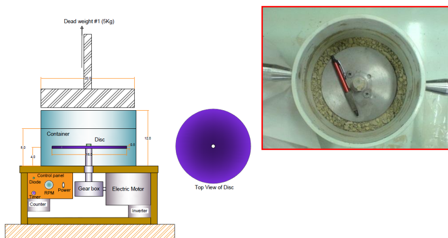
شکل ۶. نمای شماتیک دستگاه سایش ساخته شده به‌همراه نمای واقعی سنچش‌گر دیسک آهنی از بالا
