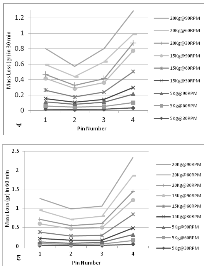
شکل ۱۴. میزان افت وزن پیچ‌ها به صورت جداگانه در حالت‌های مختلف برای زمان‌های مختلف الف) ۱۵، ب) ۳۰ و ج) ۶۰ دقیقه (از بالاترین پیچ به سمت پایین‌ترین پیچ شماره‌پین از کد ۱ تا ۴ افزایش می‌یابد)
