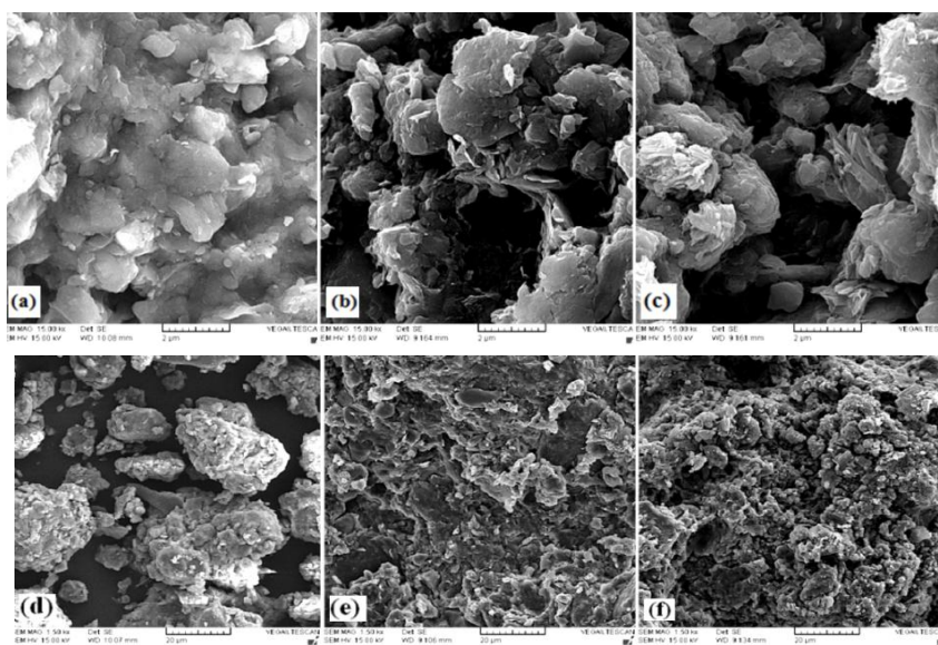
شکل ۸. عکس‌های SEM از نمونه‌های آزمایش شده (a و b) خاک رس (b و e) خاک رس با ۱ درصد آهک (c و f) خاک رس با ۳ درصد آهک
