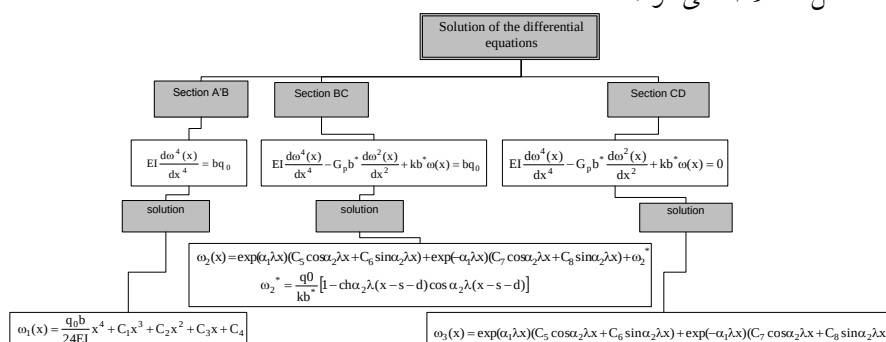
شکل ۷. فلوچارت حل معادلات دیفرانسیل جابه‌جایی قائم برای پروفیل IPE
