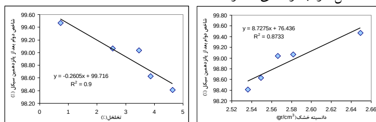
شکل ۳. ارتباط ویژگی‌های فیزیکی با شاخص دوام‌پذیری سنگ آهک‌های ایلام- سروک
