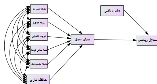
شکل ۱- مدل مفهومی رابطه میان انواع توجه، حافظه کاری، هوش سیال و دانش ریاضی با استدلال ریاضی
