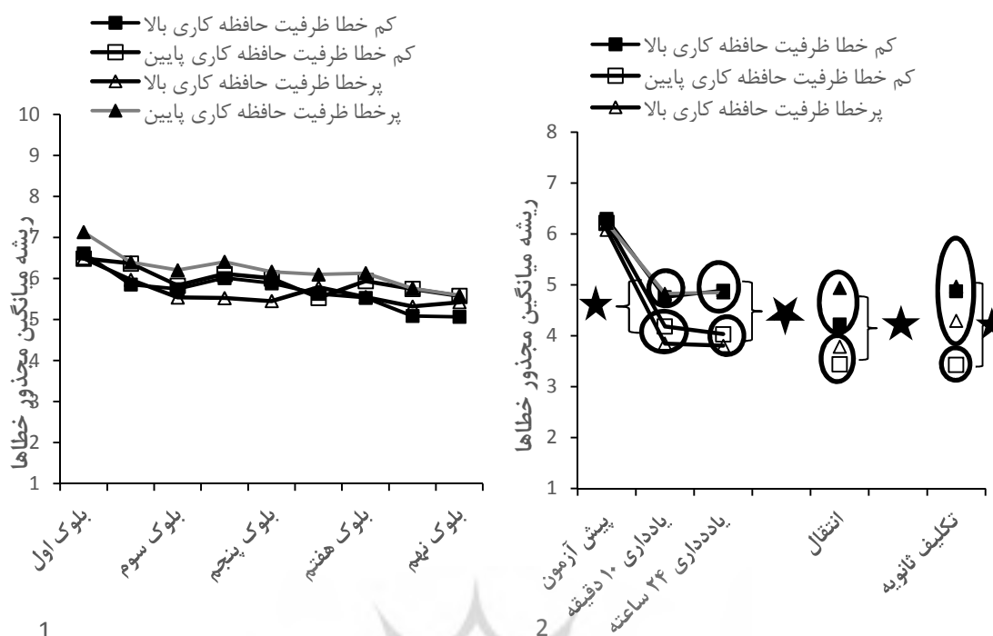
نمودار ۱ و ۲- به ترتیب مقایسه میانگین اجرای گروه‌ها در ریشه میانگین مجذور خطاها (RMSE) در بلوک‌های مرحله اکتساب و مراحل آزمایشی را نشان می‌دهد.
