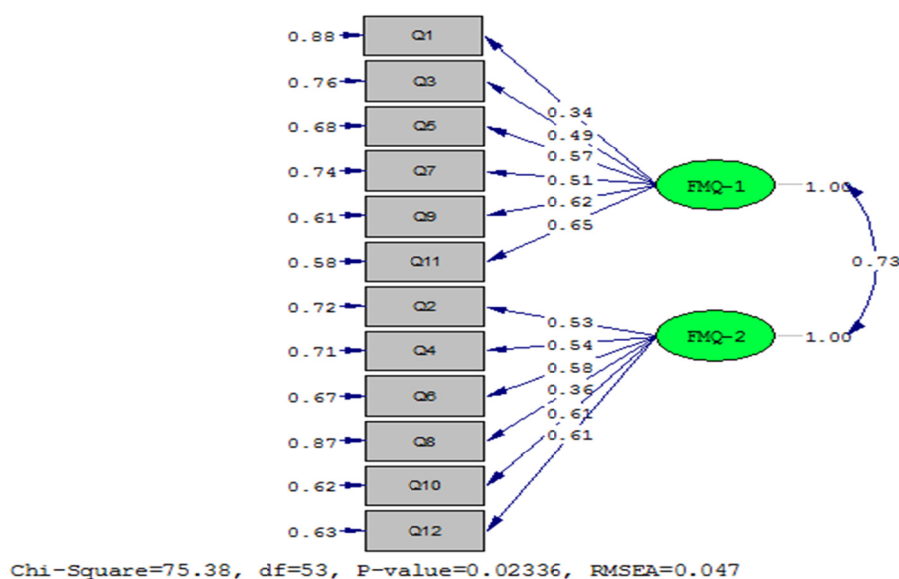
شکل ۱- نمودار تحلیل عاملی تأییدی و ضرایب مسیر پرسش‌نامه فراشناخت شناور بودن
